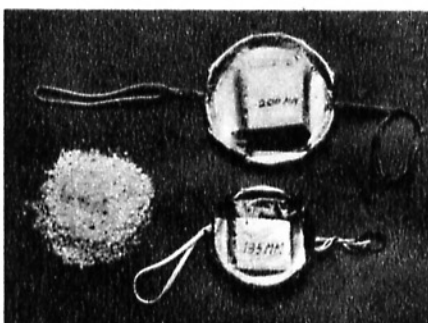
СИСТЕМА АУДИОСПУСКА В КОМПЛЕКТЕ, ВКЛЮЧАЯ ТАЙМЕР «ОЛИМПУС» И ПРОВОЛОКУ ДЛЯ ВТОРОЙ КАМЕРЫ
