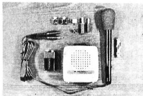
ЭТО ВСЕ НЕОБХОДИМЫЕ ДЕТАЛИ, ЧТОБЫ СДЕЛАТЬ «СПЕЦИАЛЬНЫЙ АУДИОСПУСК ХАРТЛИ» ЗА 35 ДОЛЛАРОВ
